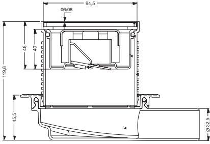
Ø 32 YAN ÇIKIŞ
